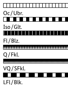
Unterbrochenes Feuer (Oc/Ubr.) Gleichtaktfeuer (Iso/Glt.) Blitzfeuer (Fl/Blz.) Funkelfeuer (Q/Fkl.) Schnelles Funkelfeuer (VQ/SFkl.) Blinkfeuer (LFl/Blk.)
